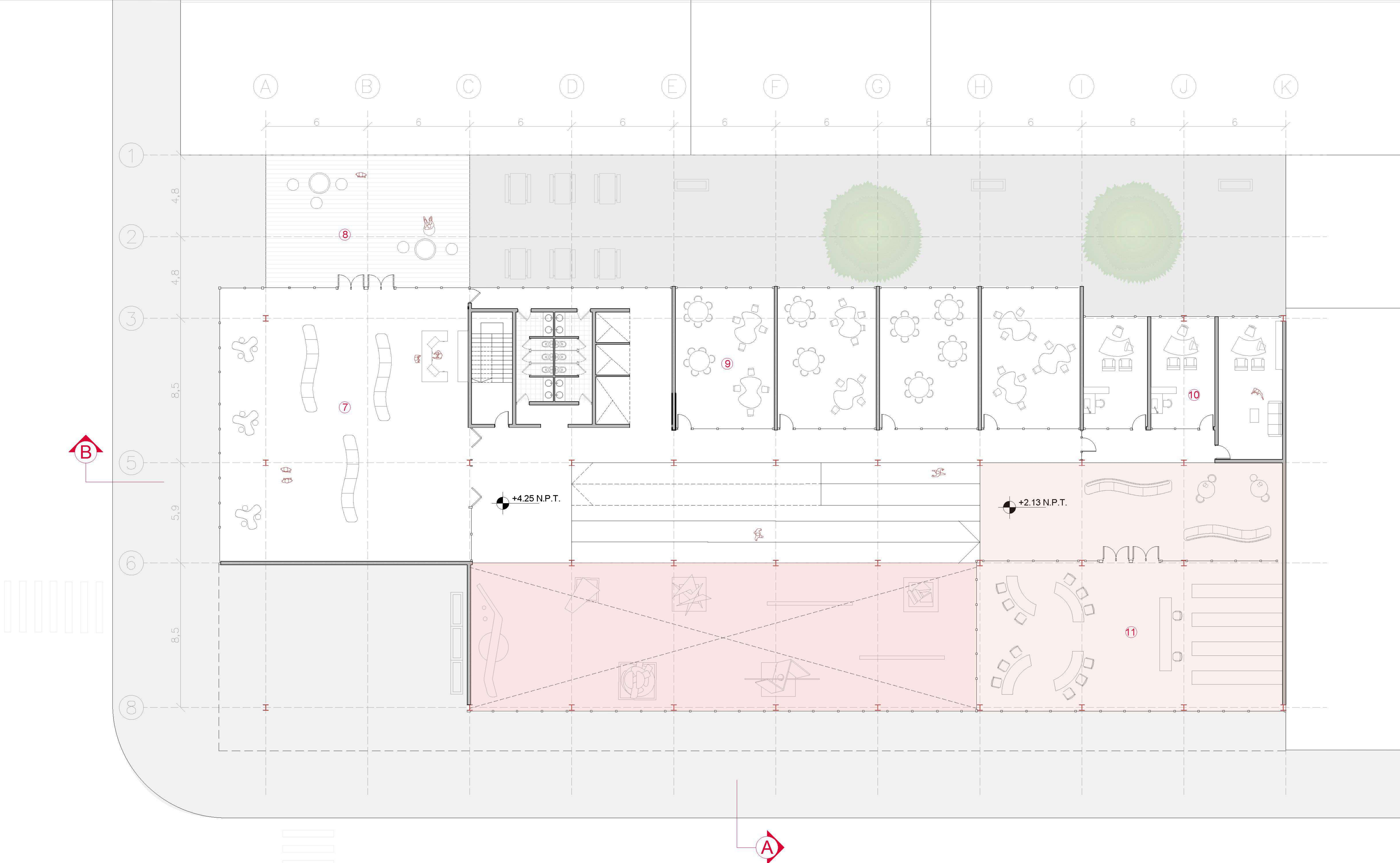
Planta 1 ESC. 1:200
