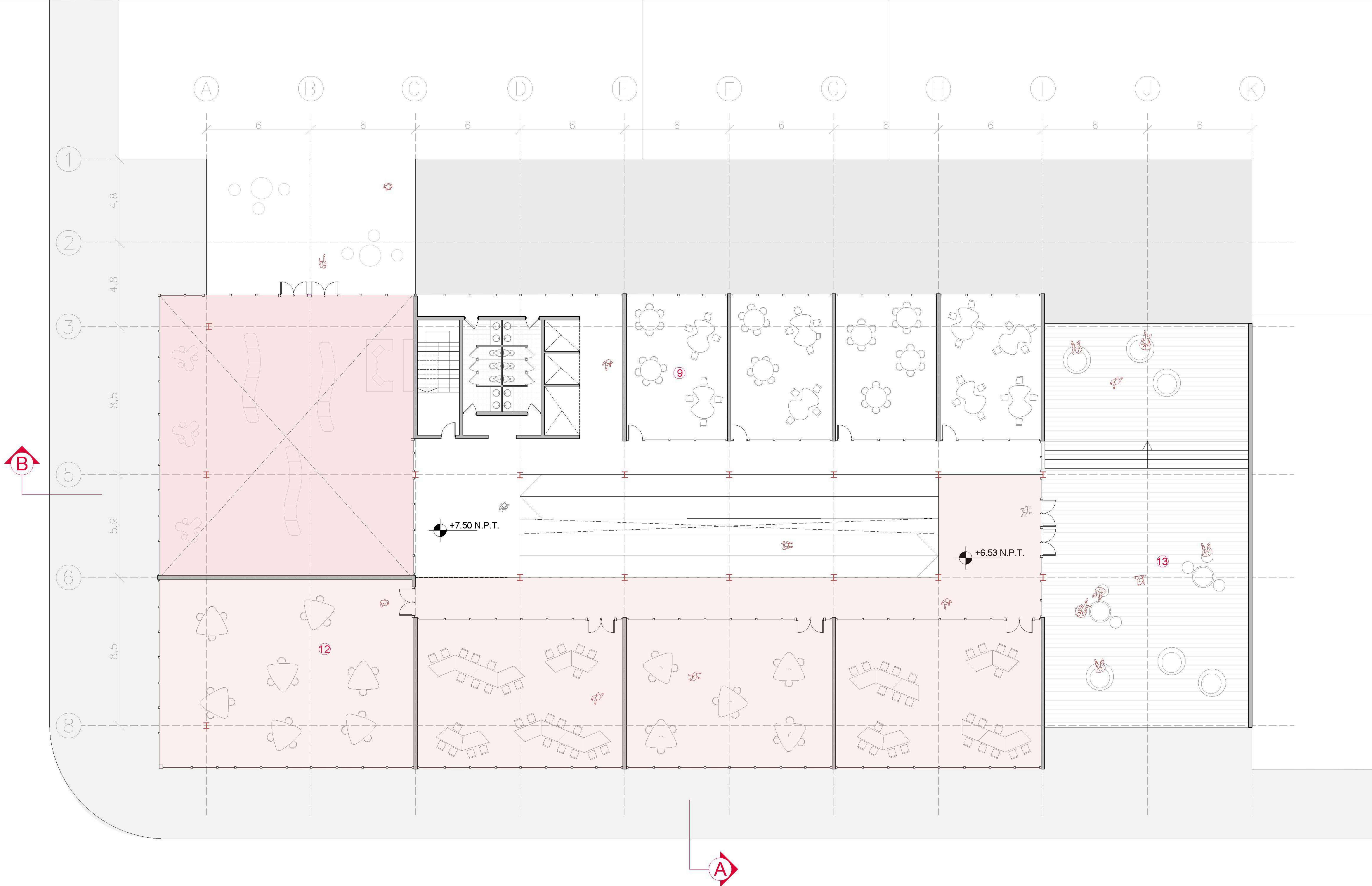
Planta 2 ESC. 1:200
